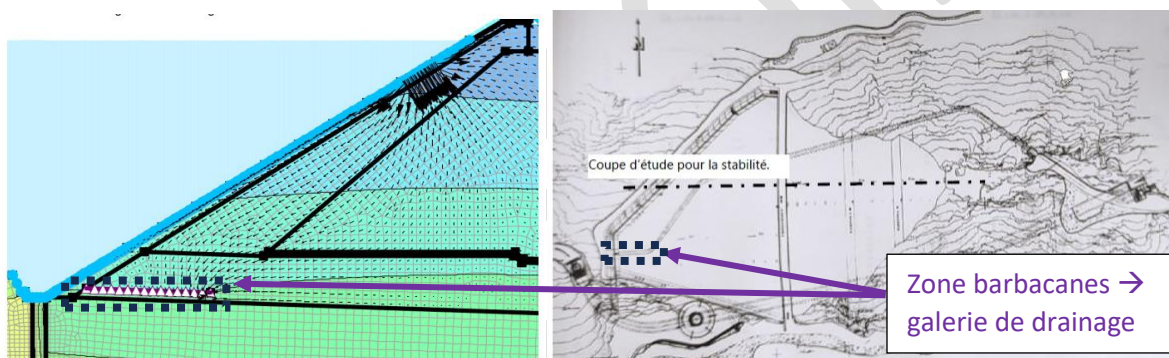
Figure 4: modélisation géoslope 2D du barrage pour une lacune d'étanchéité sur 5 m.
