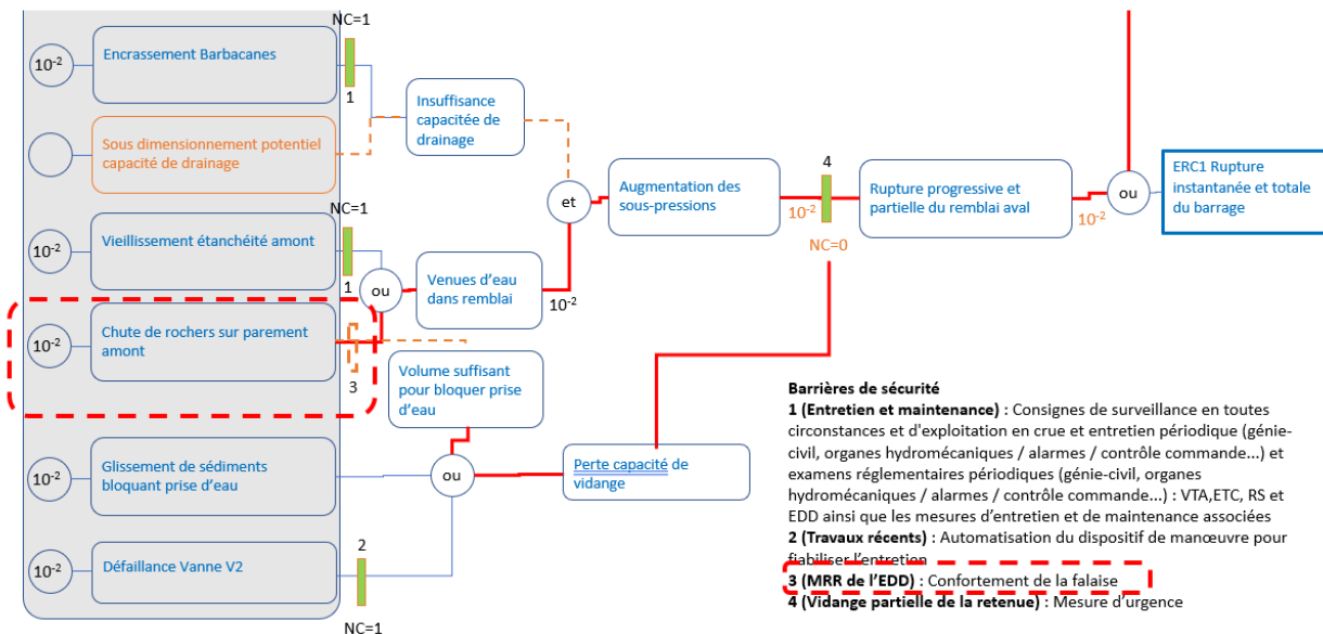
Figure 5: Arbre des défaillances pour l'évènement éboulement rocheux
