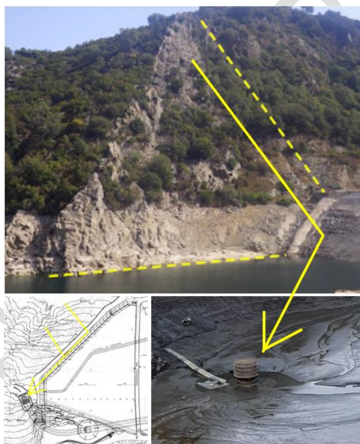
Figure 3: Trajectoires potentielles de chutes de blocs (GPA coté Rive gauche et prise d'eau au pied de la Rive droite)
