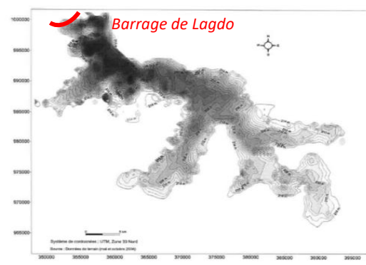
Figure 6 : Carte bathymétrique illustrant le plancher topographique de la retenue de Lagdo après la mise en eau (2004)
