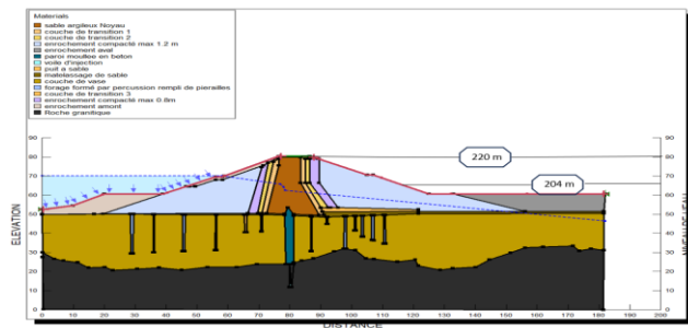
Figure 2 : Coupe transversale du barrage de Lagdo
