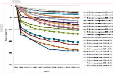
Figure 8 : Courbe de tassement du barrage
