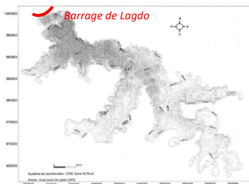
Figure 5 : Carte bathymétrique illustrant le plancher topographique de la retenue de Lagdo avant la mise en eau (1973)
