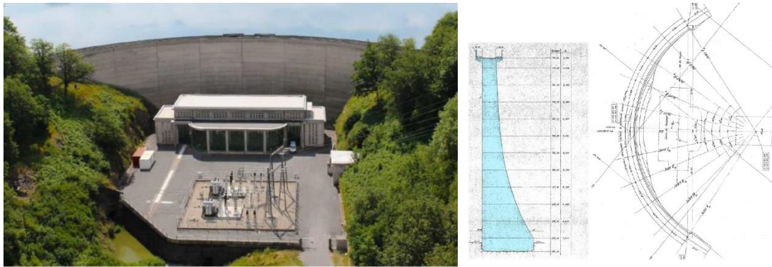
Figure 3 : Vue aval du barrage de Bage – Coupe transversale en clé et vue en plan
