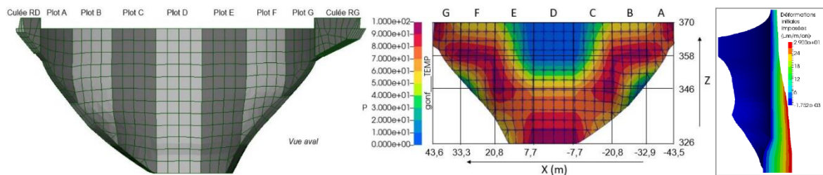
Figure 8 : Vue aval du maillage du barrage de Gour Noir – Champ thermique imposé sur le parement amont (°C) pour reproduire le gonflement des bétons (vue du barrage depuis l'amont) – Gradient amont-aval
