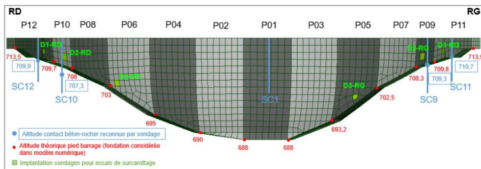
Figure 5 : Implantation des sondages carottés verticaux et des sondages horizontaux depuis le parement aval pour les mesures de contraintes par surcarottage réalisées en Octobre 2020
