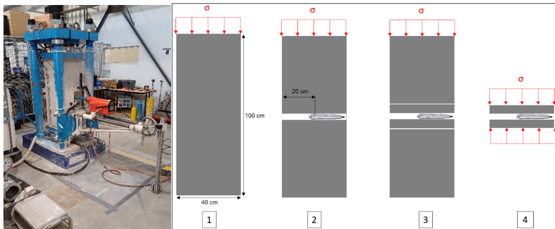
Figure 14 : Banc d'essai (presse) utilisée pour la qualification de la mesure de contrainte in-situ par surcarottage dans le béton – Phase de l'essai
