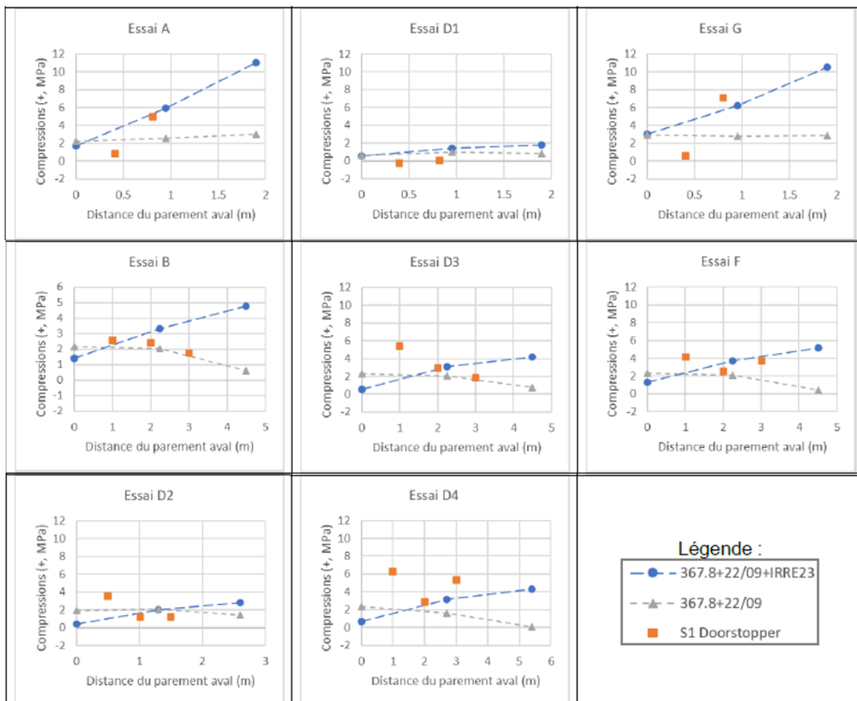
Figure 10 : Mesure de contraintes au barrage de Gour Noir en fonction de la profondeur depuis le parement aval comparées avec les contraintes en parement du modèle numérique sans et avec prise en compte des effets irréversibles
