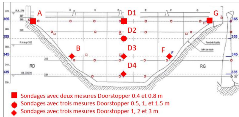
Figure 9 : Positionnement des sondages pour les mesures Doorstopper sur le barrage de Gour Noir
