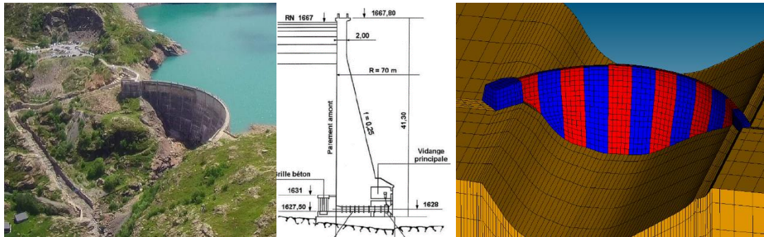
Figure 11 : Barrage des Gloriettes vu depuis l'aval – Profil central du barrage – Maillage utilisé pour l'étude de comportement
