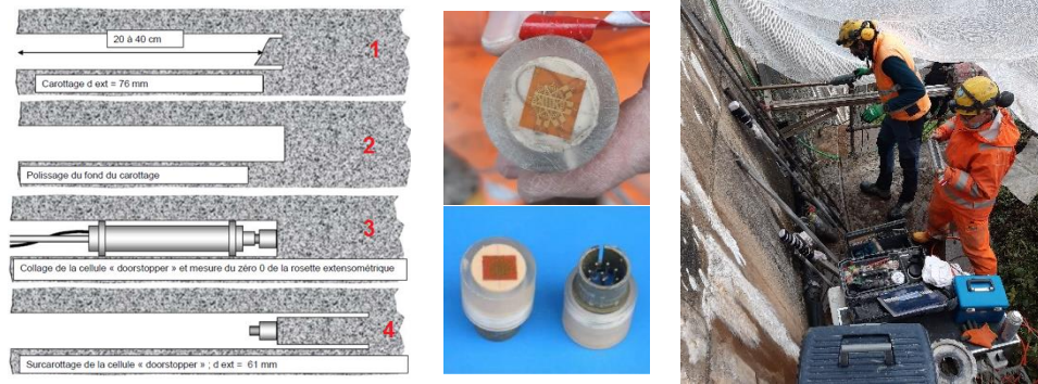
Figure 1 : Principe de la mesure de surcarottage avec cellule Doorstopper
