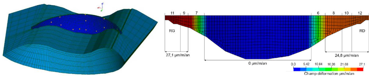
Figure 4 : Maillage du barrage de Bage – Champ de déformation imposé ( \mu\text{m}/\text{m}/\text{an} ) pour le calage des déplacements irréversibles (vue du barrage depuis l'amont)
