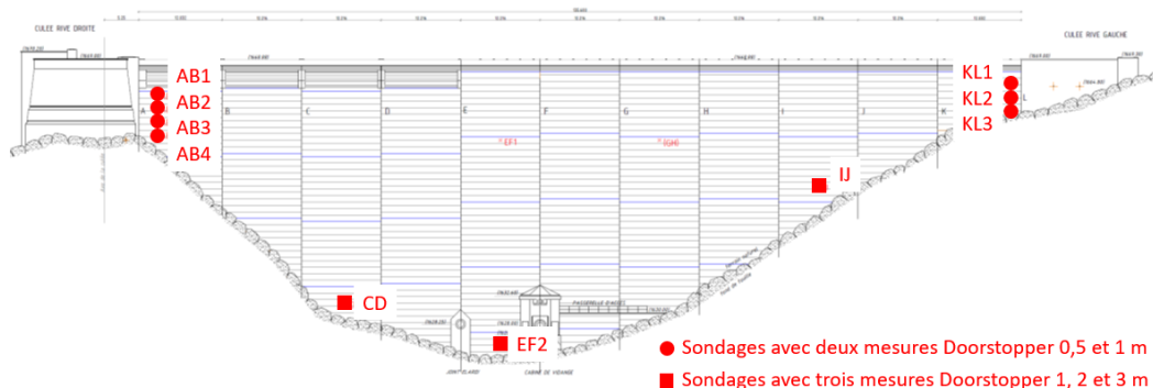
Figure 12 : Emplacement des sondages pour les surcarottages et nombre d'essai par sondage
