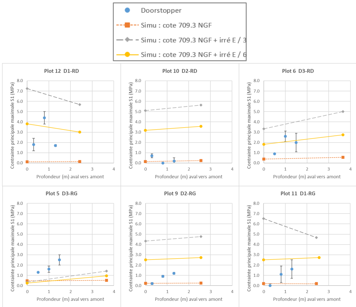
Figure 6 : Mesure de contraintes au barrage de Bage (Doorstopper) en fonction de la profondeur depuis le parement aval comparées avec les contraintes en parement du modèle numérique sans (orange), avec (gris et jaune) prise en compte des effets irréversibles pour deux modules long-terme – Simulation avec module long terme / 6 retenue
