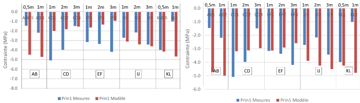
Figure 13 : Comparaison de la contrainte principale majeure calculée par le modèle numérique, avant (haut) et après (bas) recalage du modèle, avec celle mesurée in-situ
