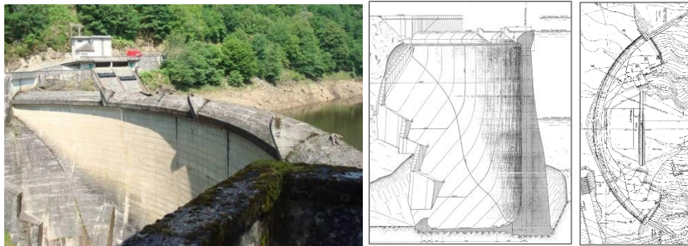
Figure 7 : Barrage de Gour Noir vu depuis la culée RG – Profil central du barrage – vue en plan
