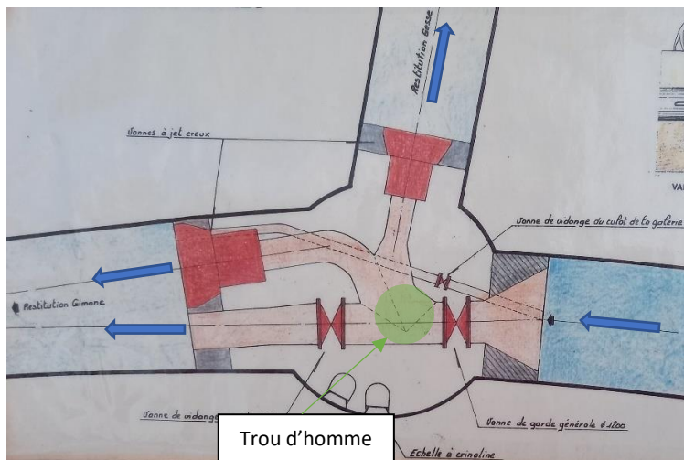
Figure 6 : Chambre des vannes du barrage de la Gimone
