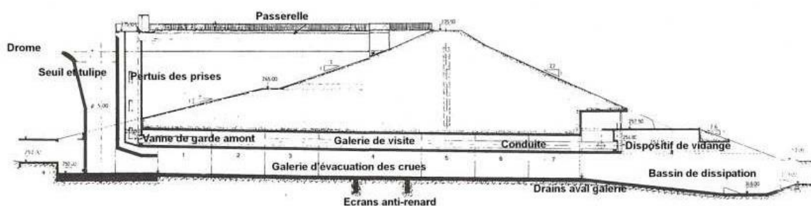
Figure 8 : Schéma de principe du barrage – Profil dans l'axe de l'évacuateur de crues et de la vidange
