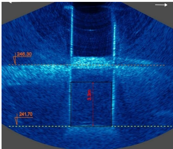
Figure 4 : Vue d'ensemble de la prise d'eau – image acoustique
