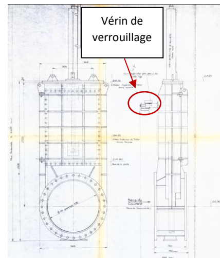
Figure 7 : Vanne de garde
