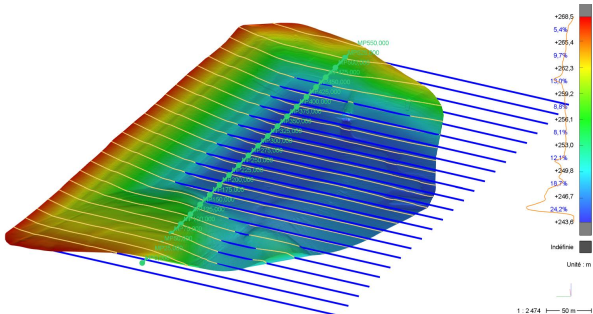
Figure 3 : Relevé bathymétrique du parement amont du barrage de la Gimone
