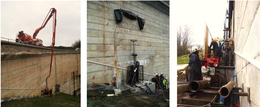
Figure 5 : Réalisation d'un nouveau pendule au niveau de la culée RD d'un barrage voûte (Monceaux)
