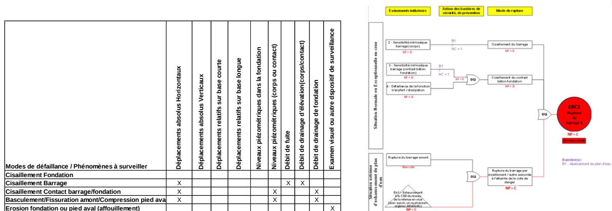
Figure 8 : Exemple de tableau de pertinence de phénomènes à surveiller d'un barrage poids (à gauche) élaboré en cohérence avec l'analyse de risque rupture barrage de l'EDD (à droite)
