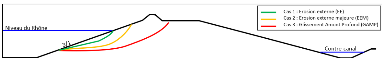
Figure 2 : Profils d'études pour le glissement amont
