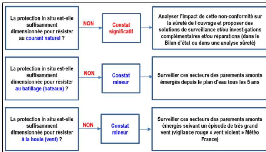
Figure 8 : Classification des constats issues du diagnostic des protections en enrochements
