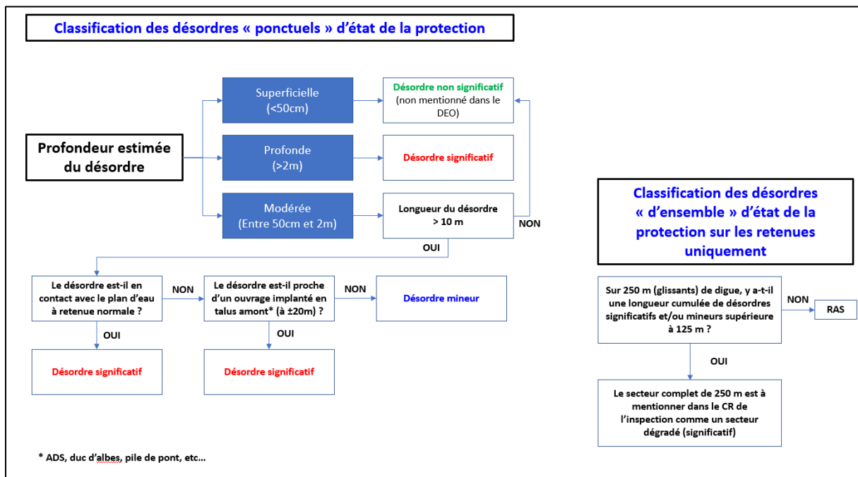
Figure 5 : Classification des désordres d'état de la protection
