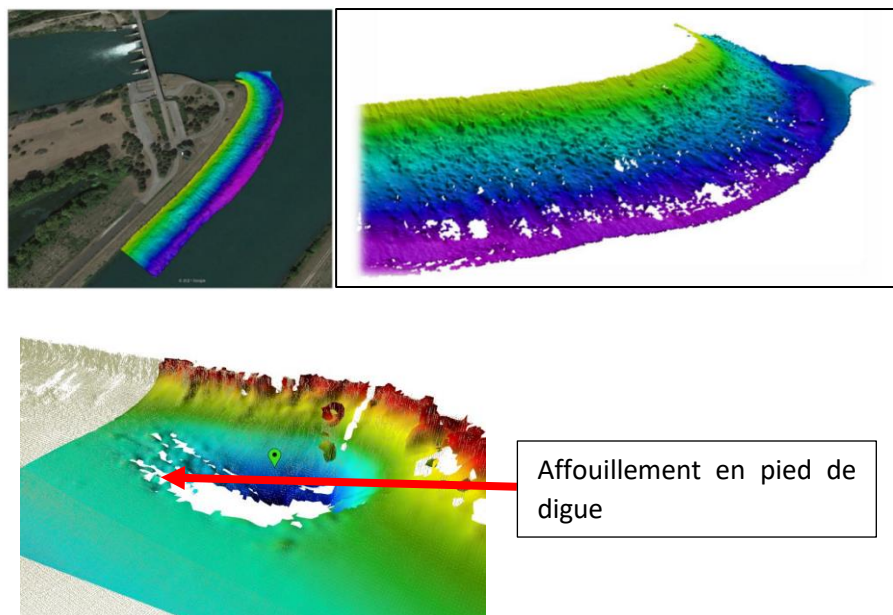
Figure 6 : Modèle 3D issue d'un levé bathymétrique sur l'aménagement de Saint-Vallier (vue des enrochements)
