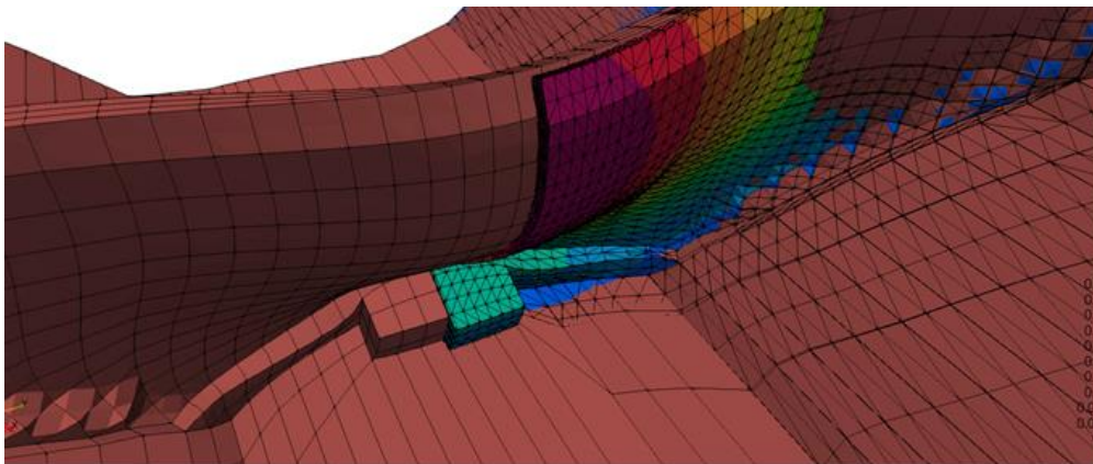
Figure 17 - Comparaison des déplacements de la voûte en configuration initiale (en rouge) et avec modélisation de la fosse et d'une diaclase (en couleur et en coupe) - Vue d'aval
