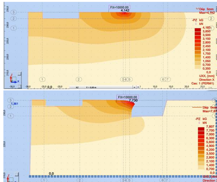
Figure 14 - Modèle 2D de la fondation avec (bas) et sans (haut) fosse d'érosion, l'empreinte côté gauche correspond à la fouille du barrage, celle de droite à la fosse d'érosion.
