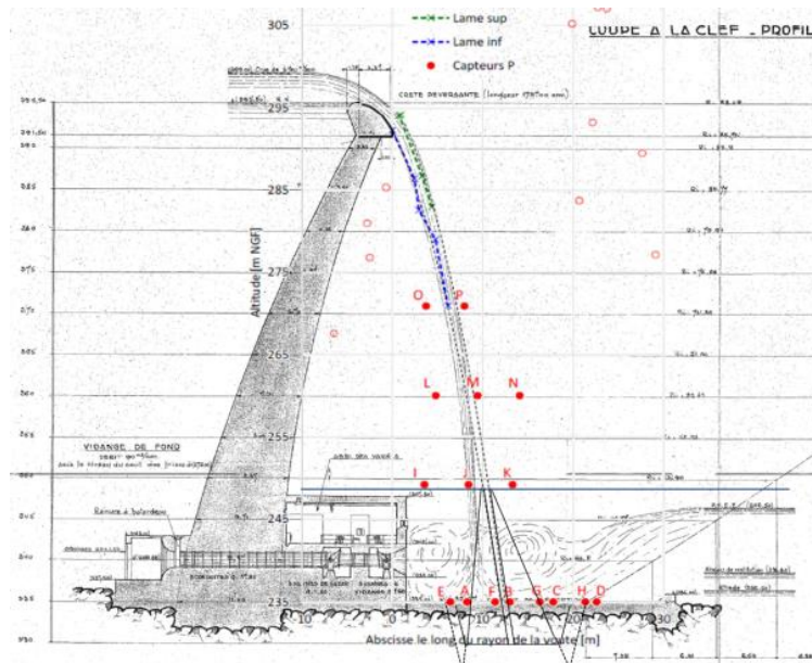
Figure 13 - Géométrie de la fosse d'érosion théorique
