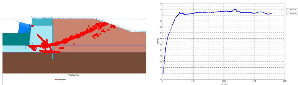
Figure 9: points plastiques délimitant la surface de rupture d'après la méthode « C-Phi réduction » ; évolution du déplacement du point de référence en fonction du facteur de réduction appliqué aux résistances mécaniques « C-Phi réduction »
