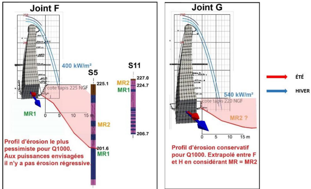
Figure 5 - Érosion vue des joints F et G à ZQ1000, coupes issues de l'étude spécifique d'érodabilité
