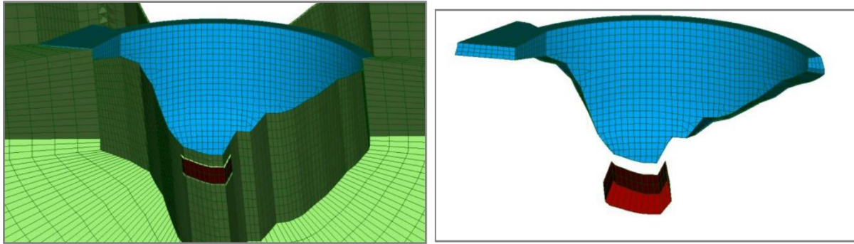
Figure 11 - Modèle numérique du barrage « C » et position de la fosse d'érosion aval.
