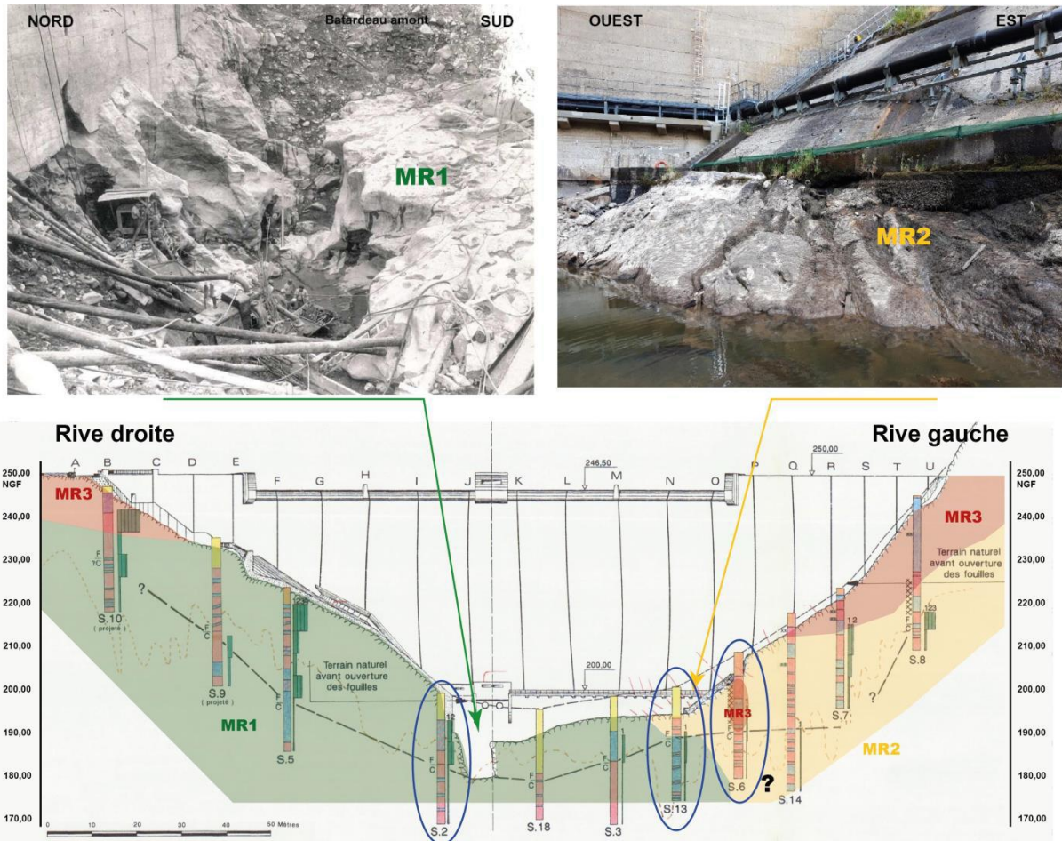
Coupe au pied aval de la fondation (assumant le fait que le barrage est fondé sur le rocher compact)
