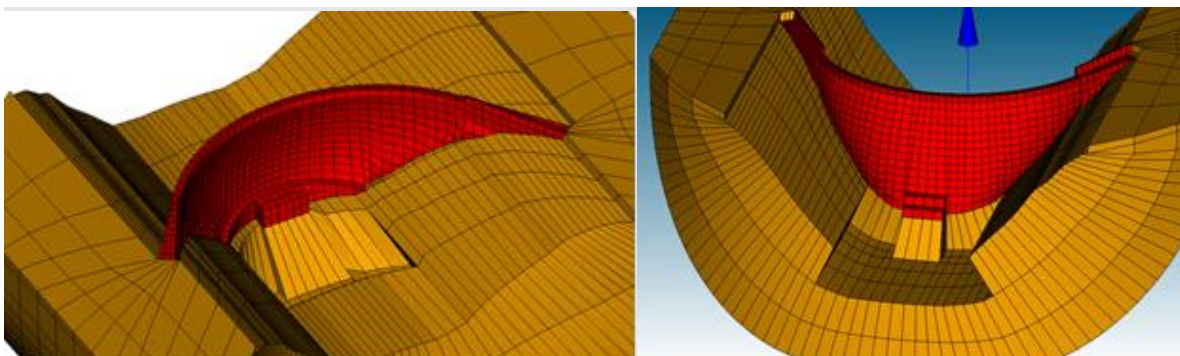
Figure 15 - Gauche : Modélisation d'une fosse en pied aval – Droite : Modélisation d'une diaclase en pied amont
