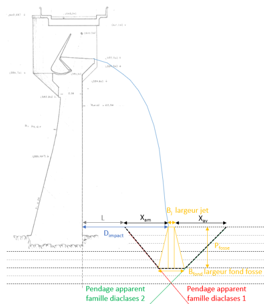
Figure 2 – Exemple de détermination de fosse d'érosion selon l'angle de diffusion du jet et le pendage du rocher
