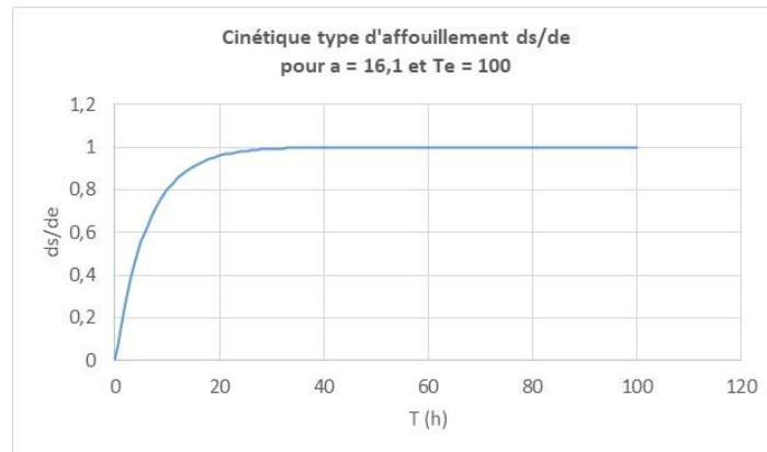
Figure 1 – Exemple de courbe de cinétique d'affouillement selon Spurr
