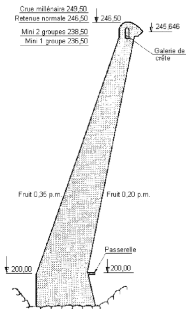
Figure 3 - Vue en coupe du barrage « A »
