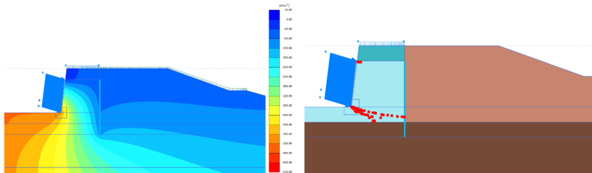
Figure 8: Isovaleurs de sous pressions estimées dans le rocher en tenant compte du drainage et du zonage des matériaux (rocher superficiel altéré par les tirs en bleu clair, rocher superficiel non altéré en brun clair, rocher sain en brun foncé)
