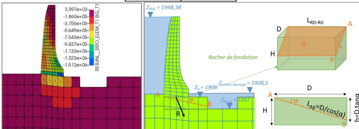
Figure 12 - Compressions sur une coupe centrale du modèle numérique, cas PHE (gauche). Plan de cisaillement considéré pour la vérification de la stabilité de la fondation du barrage après création d'une fosse d'érosion (droite)
